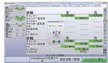
スポイラーモードによる測定画面
