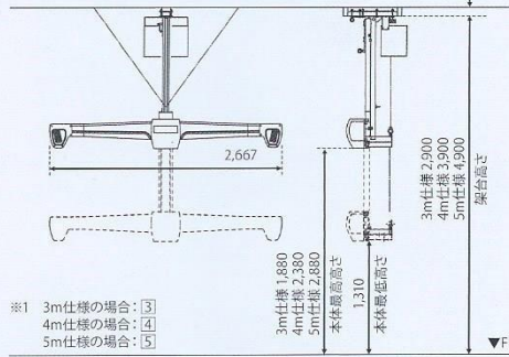
③ 吊り下げ昇降タイプ WA670-HE421RC (※1)
