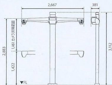
① 支柱タイプ (電動昇降付) WA670-HE421L
