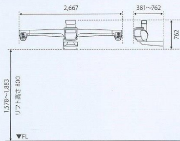
② 壁・吊りタイプ WA670-HE421W
